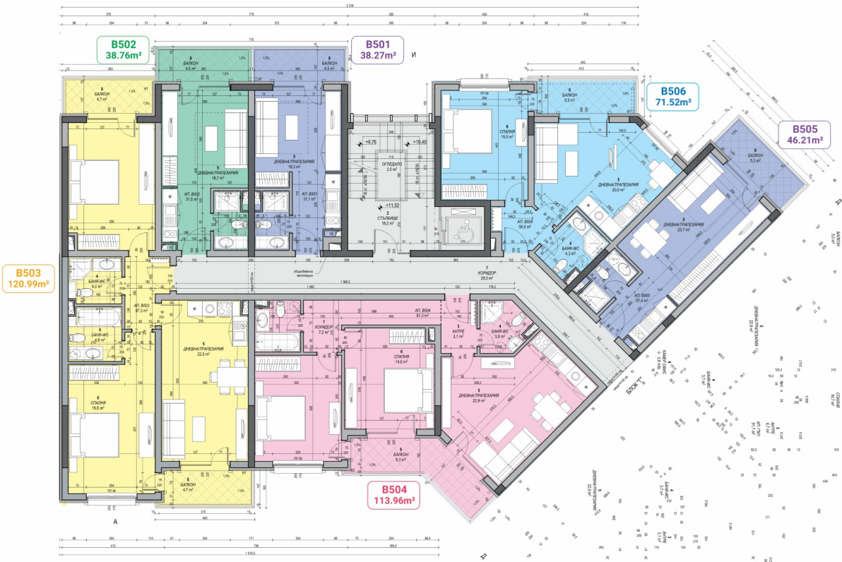
Разпределение на етажа +11.52 / Блок В / М 1:50
